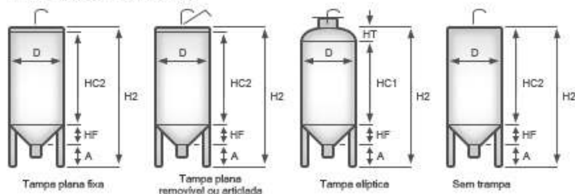
Tanque vertical fundo cônico
